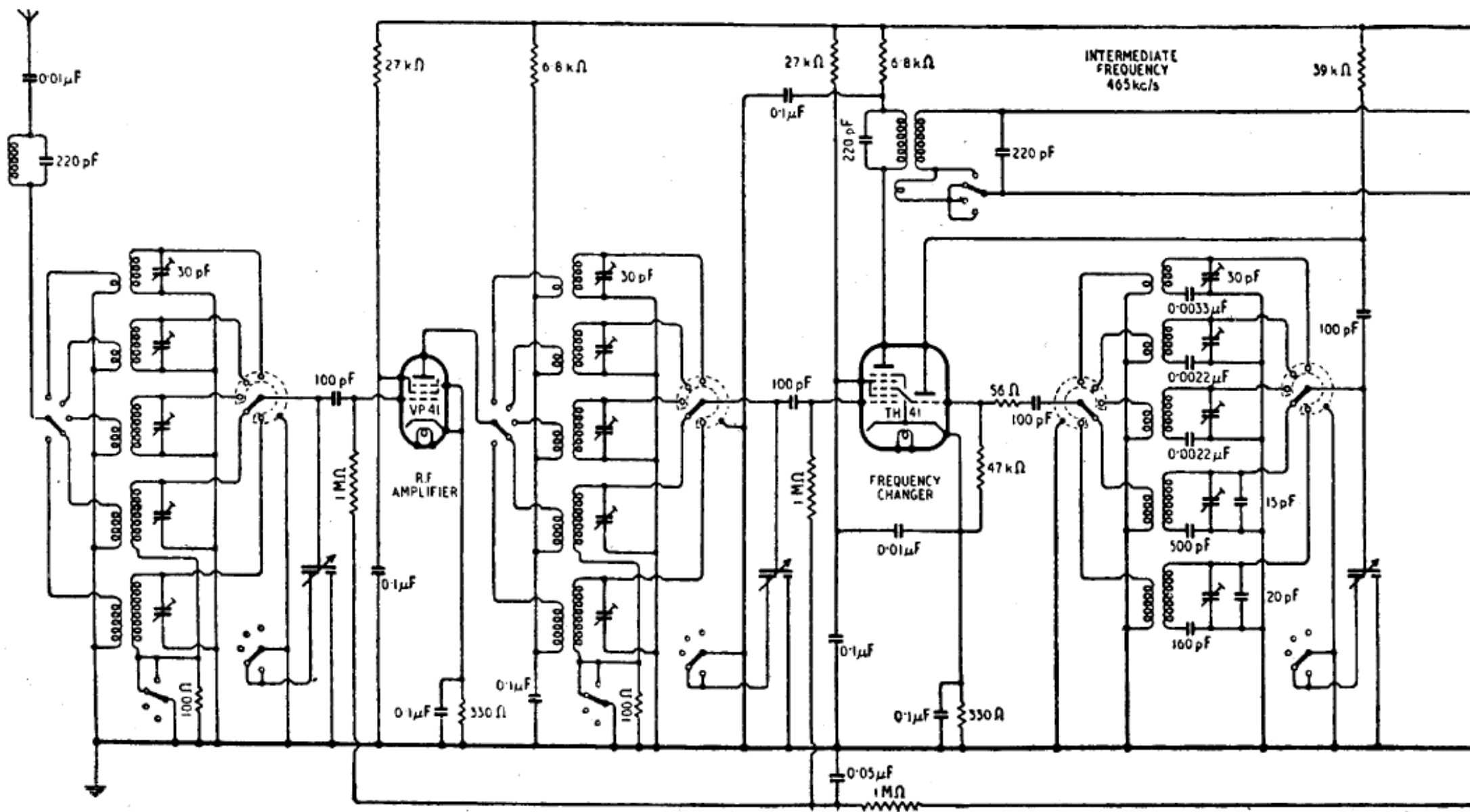
Parte AF della supereterodina R.G.D. 1046 G.
